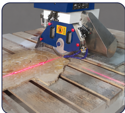
Láseres de alineación.
